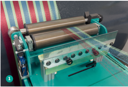
Sectional warping 分条整经
