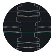
Symm-Net花边
