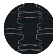
Symm-Net
